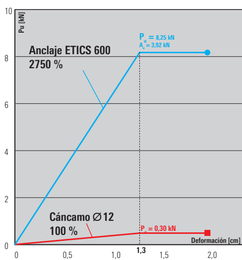
Comparación entre el cáncamo y el anclaje ETICS
