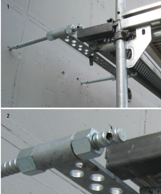
1 Uso del anclaje ETICS con en andamio Blitz. 2 Rápido montaje y desmontaje gracias al travesaño de anclaje perforado.
